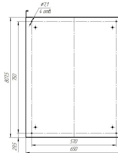
Рисунок 2 – Установочные размеры СТС-504ВК
