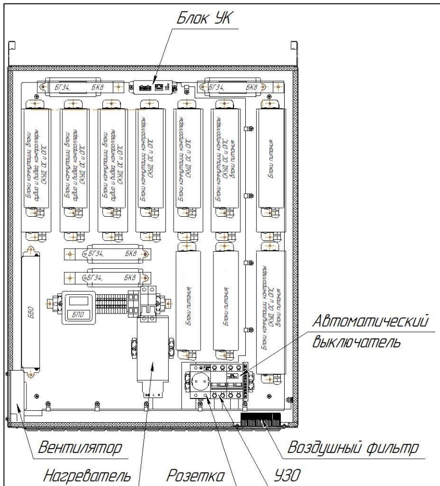
Рисунок 1 – Размещение блоков на монтажной панели
