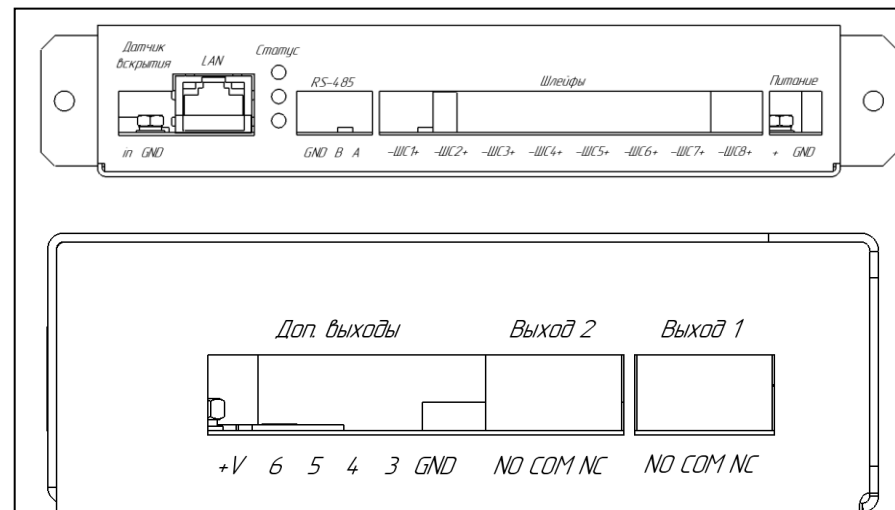
Рисунок 1 – Назначение разъемов контроллера
