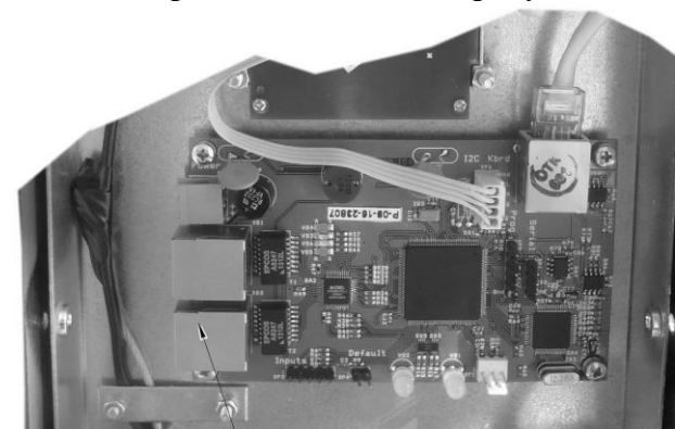
Подключение сети Ethernet+PoE
