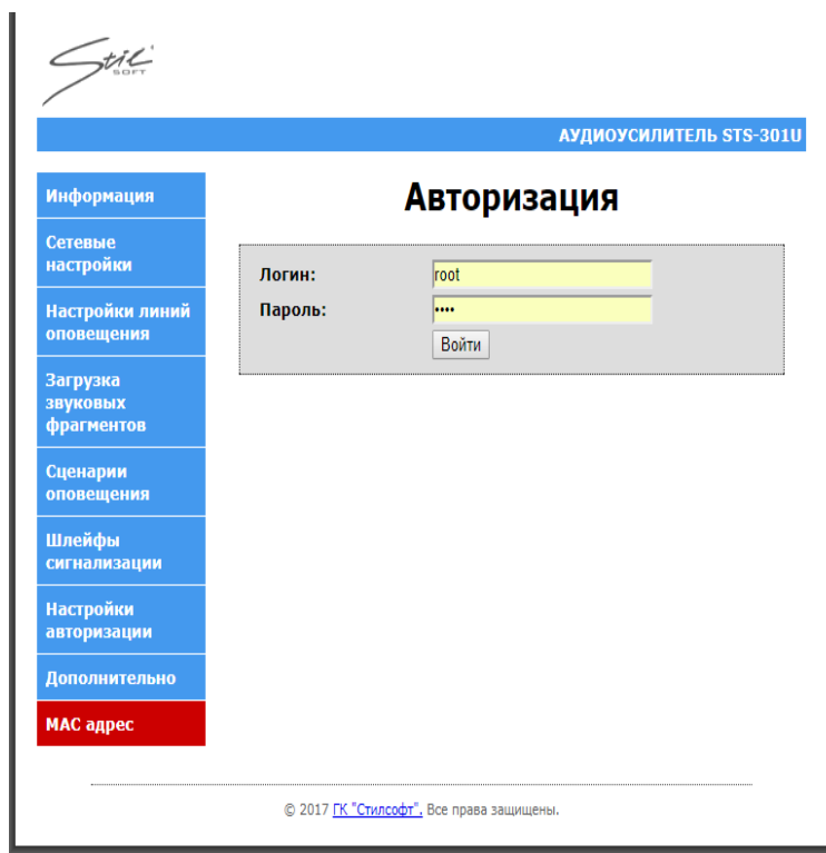
Рисунок 7 – Окно авторизации
